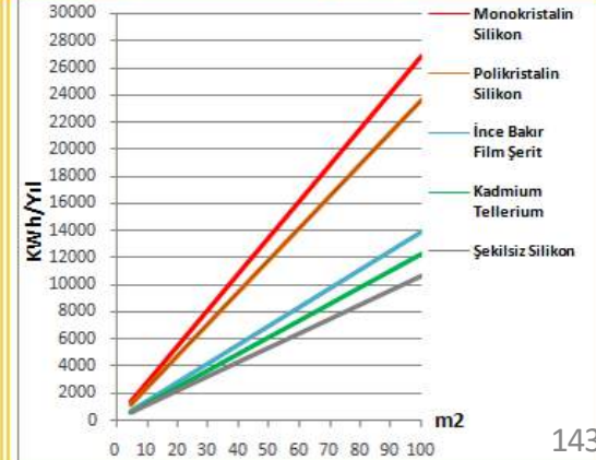
MUĞLA PV Tipi-Alan-Üretilebilecek Enerji (KWh-Yıl)
