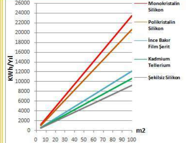
RİZE PV Tipi Alan Üretililecek Enerji (KWh-Yıl)
